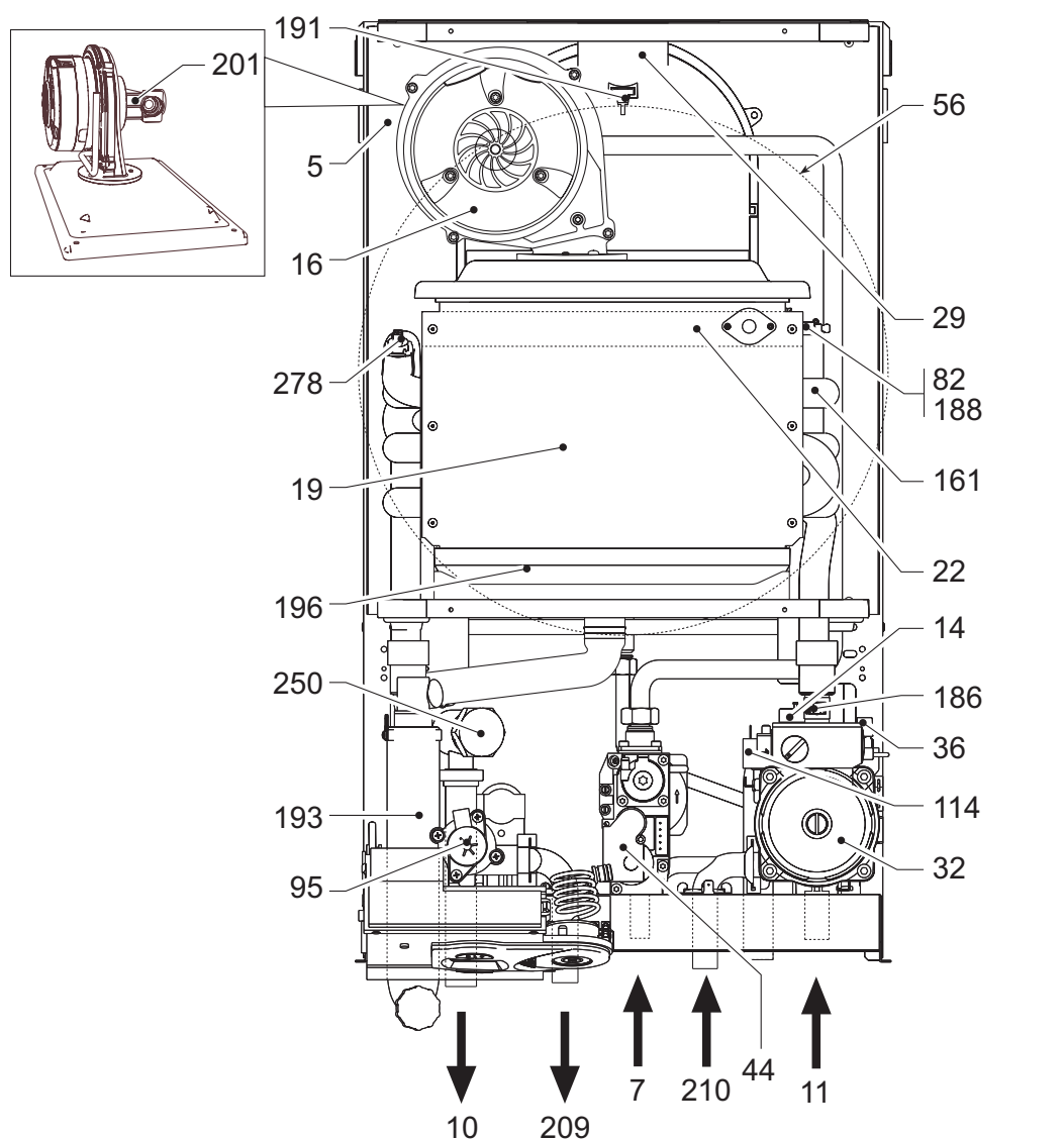
fig. 29 - Vue générale
