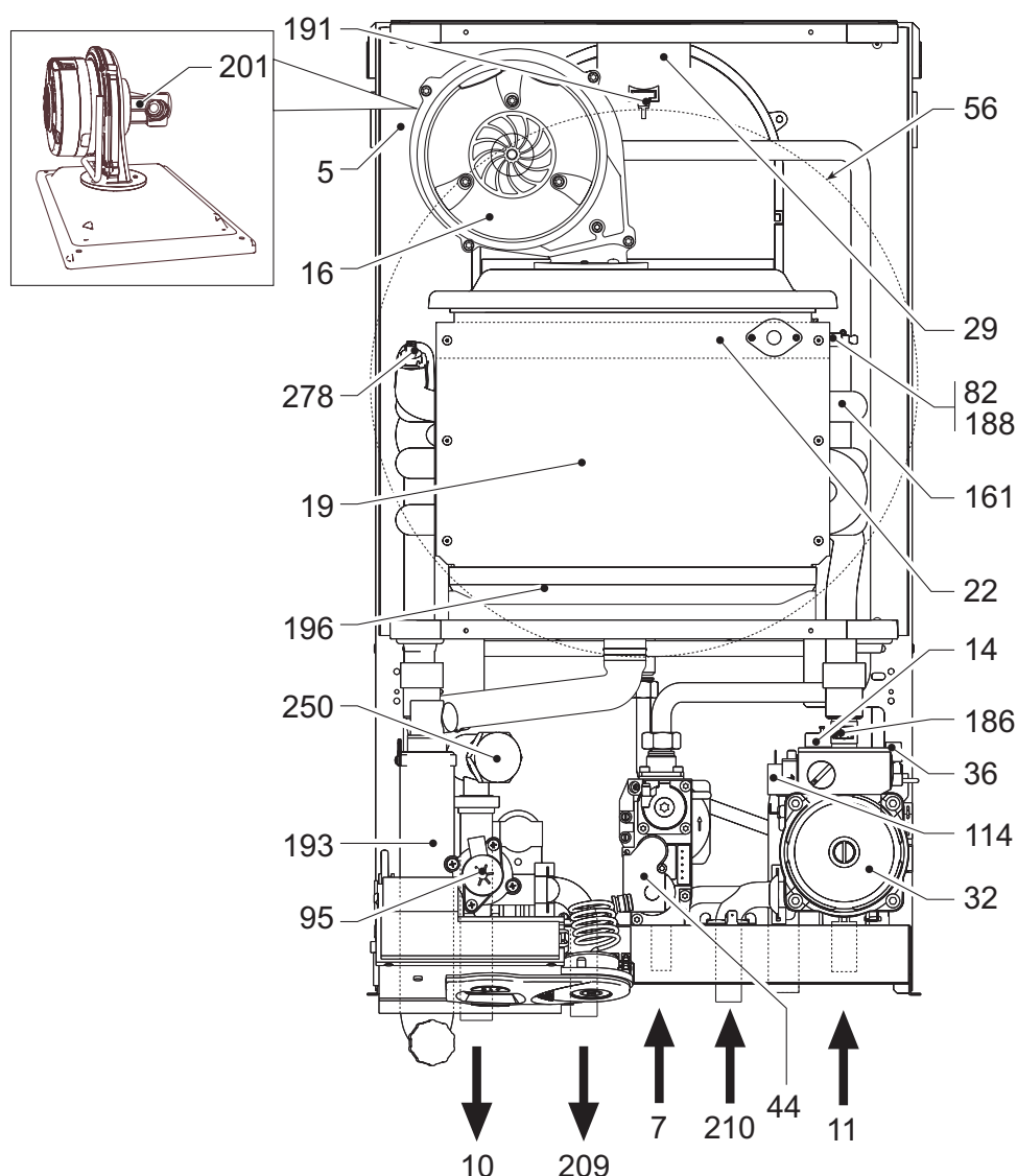
fig. 29 - Aanzichttekening
