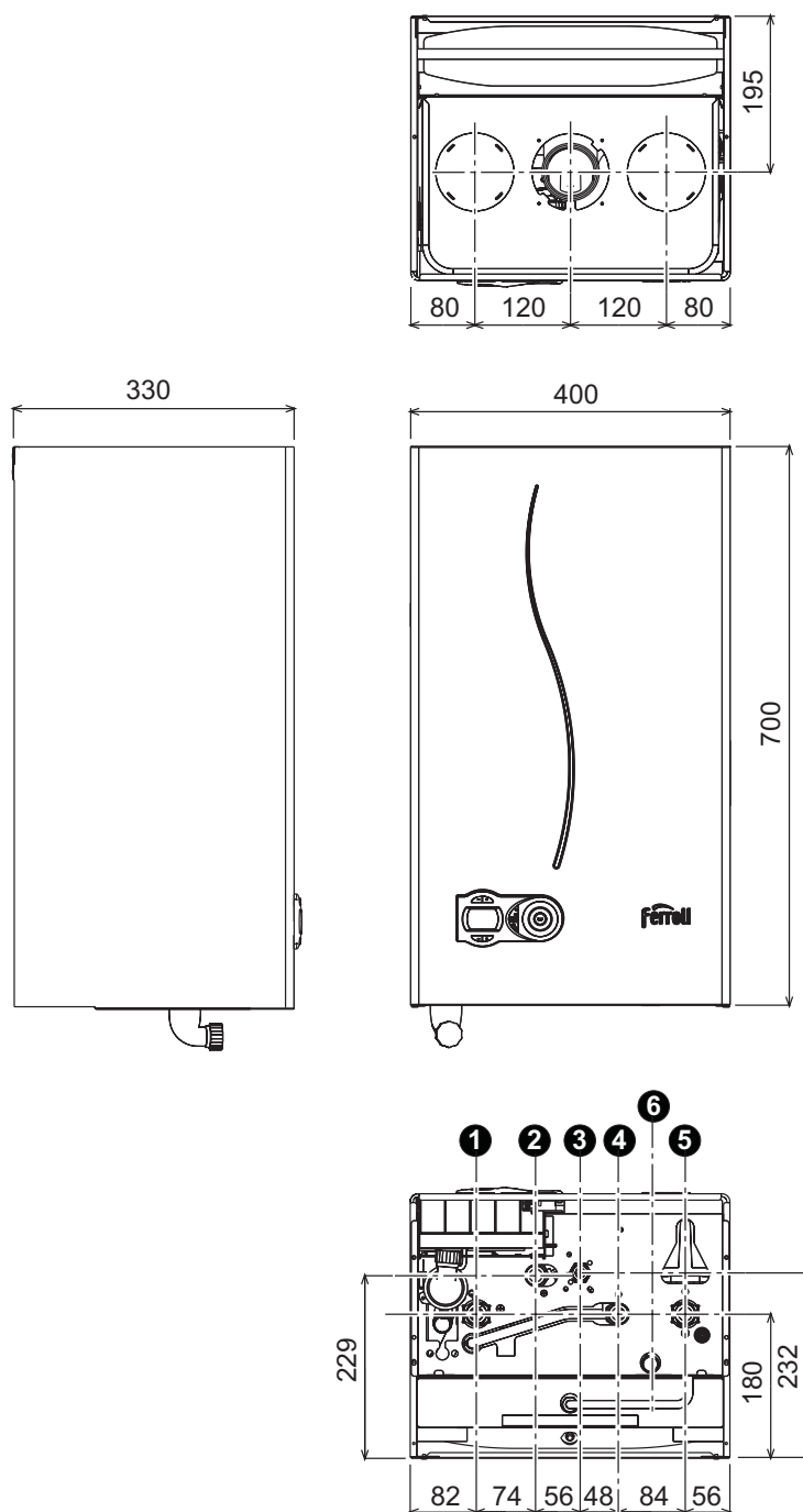
fig. 28 - Afmetingen en aansluitstukken
