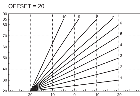
fig. 13 - Exemple de déplacement parallèle des courbes de compensation
