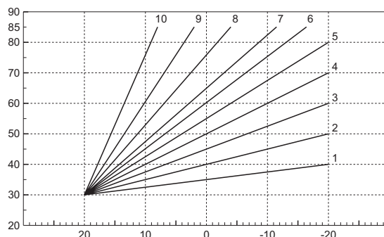
fig. 12 - Compensatiecurven
