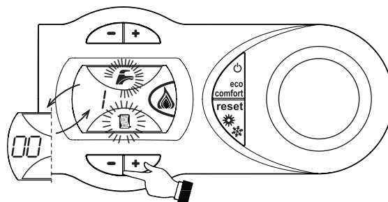
fig. 25 - TEST-modus (verwarmingscapaciteit = 100%)
