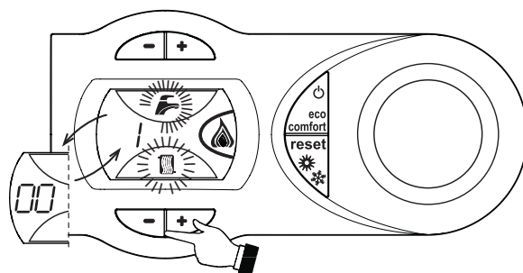
fig. 25 - Modalité TEST (puissance chauffage = 100%)
